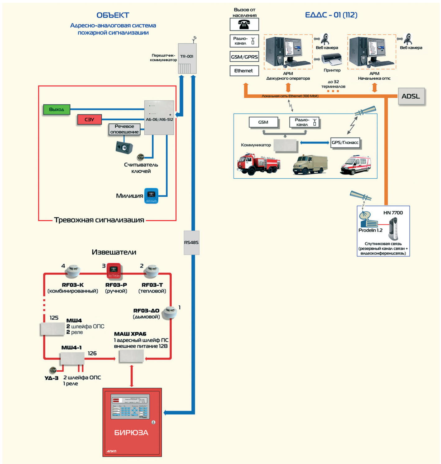
Рис. 1 Структурная схема системы противопожарного мониторинга "Горизонт-нт"
